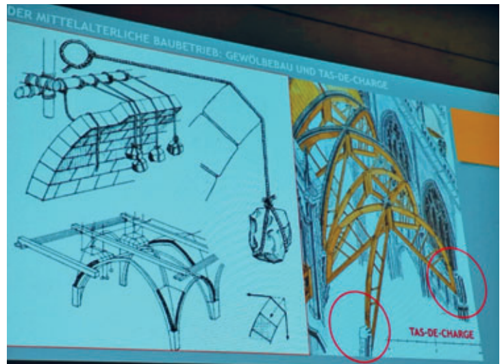
Erläuterungen zum Gewölbebau
